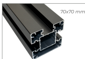
GF001 HLINÍKOVÝ SLOUPEK
